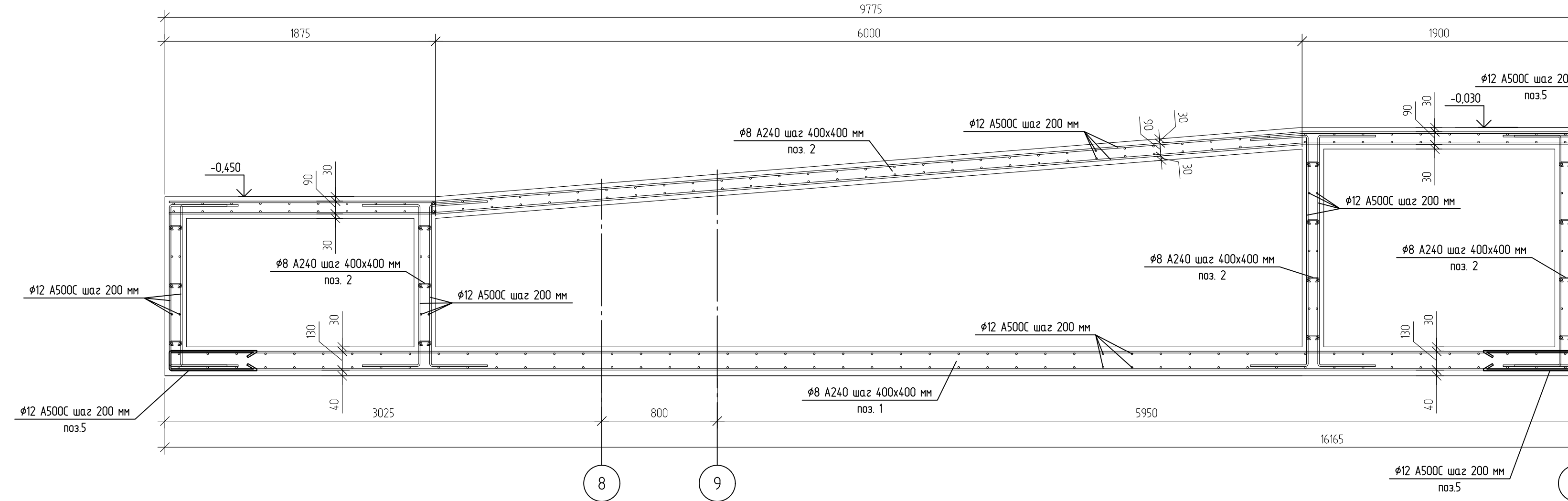
Схема армирования колонны Разрез 5-5
