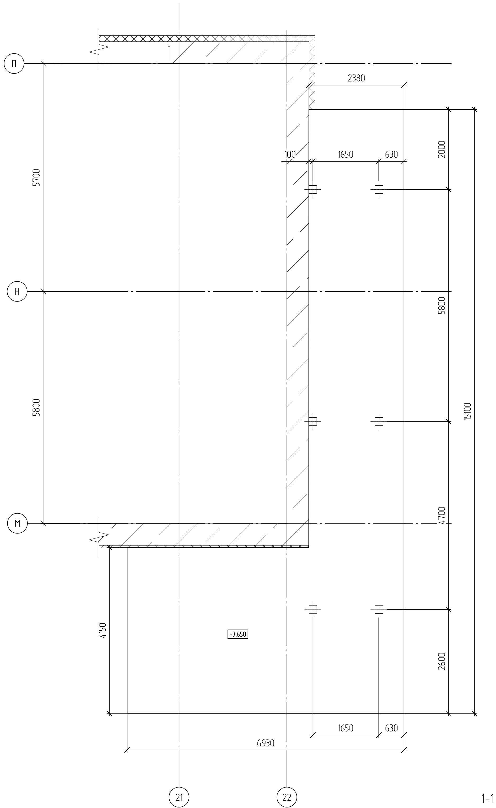
Схема плиты покрытия ПП-1 на отм. +3,650
