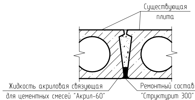
Схема заделки трещин в плитах перекрытия
