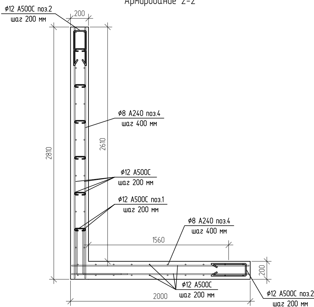
Армирование 2-2
