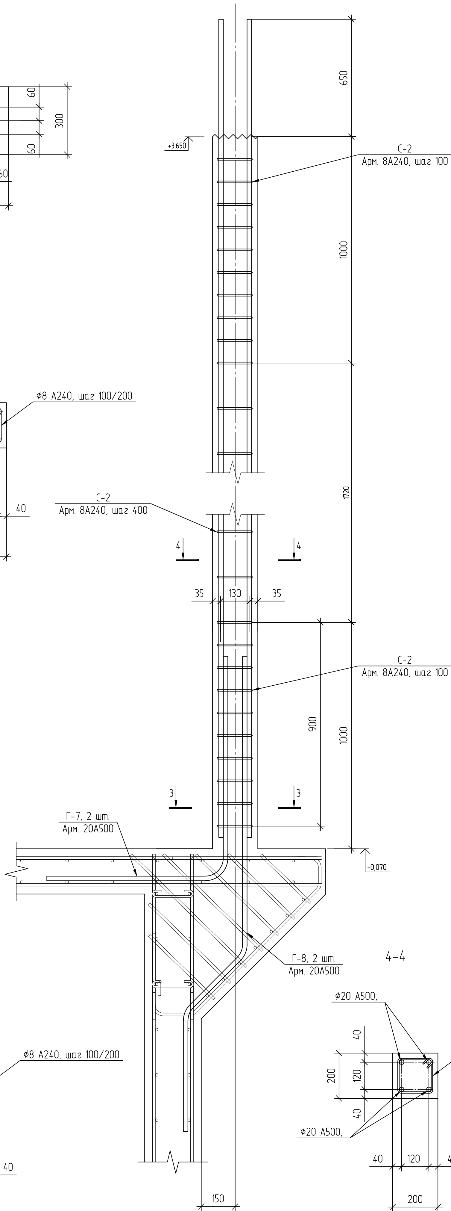
Колонна К-2
