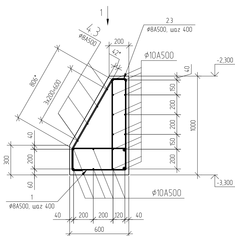
А-А
