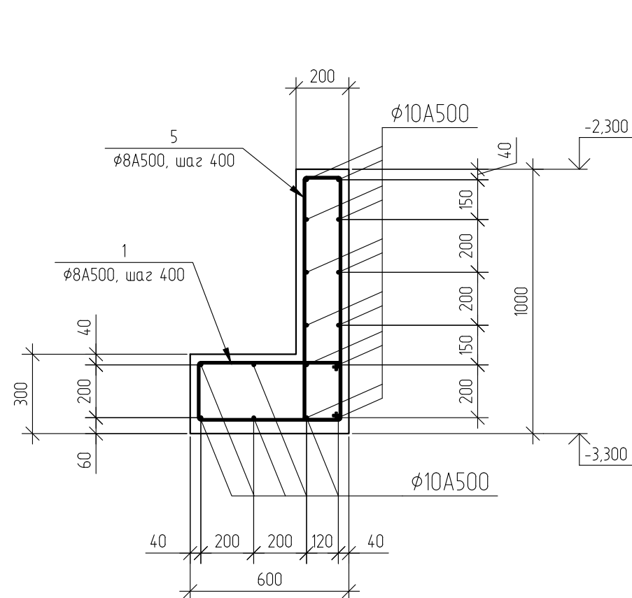
Б-Б
